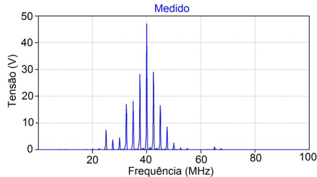
Figura 9. Gráfico no domínio da frequência do sinal captado pela antena receptora.
