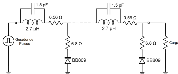
Figura 3. Modelo LT-SPICE da LTNL.
