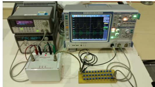
Figura 5. Foto do Setup de Medição.
