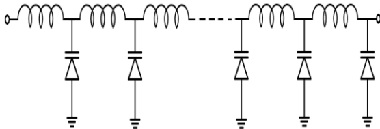
Figura 1. LTNL com varactores e indutores.
