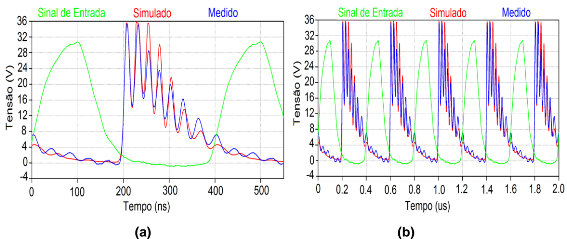
Figura 6. Gráficos no domínio do tempo dos sinais de entrada (medido) e saída da LTNL na carga de 470 \Omega (simulado e medido) mostrando 1 pulso (a) e 5 pulsos (b).
