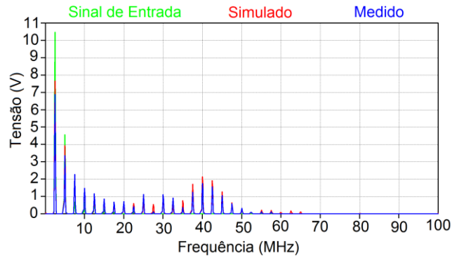
Figura 7. Gráfico no domínio da frequência dos sinais de entrada (medido) e saída da LTNL na carga de 470 \Omega (simulado e medido).
